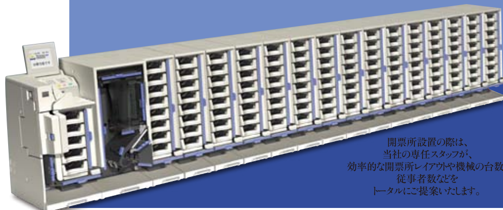
増設ユニット15台 (125段スタッカー) および天地表裏反転ユニット接続例
